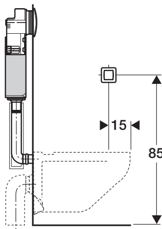
Misure di montaggio del comando pneumatico manuale posato lateralmente
