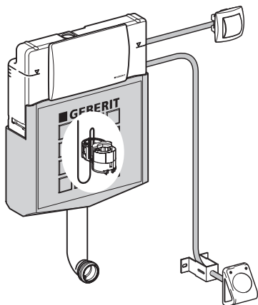
Cassetta di risciacquo da incasso con comando pneumatico manuale e a pedale
